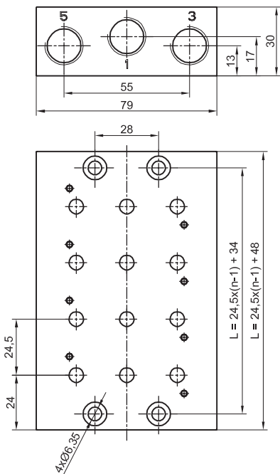
PŁYTA PRZYŁĄCZENIOWA DO ZAWORÓW ZMG 5/2 G1/8
