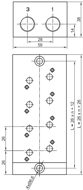
PŁYTA PRZYŁĄCZENIOWA DO ZAWORÓW ZMG 5/2 G1/4
