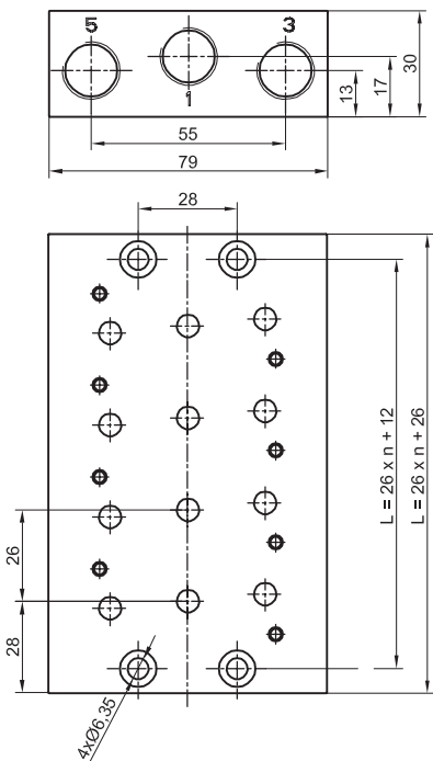
PŁYTA PRZYŁĄCZENIOWA DO ZAWORÓW ZMG 5/2 G1/4
